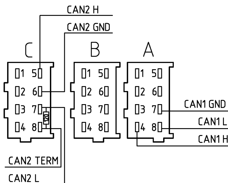
Рисунок Г.6 – Подключение CAN-шины
